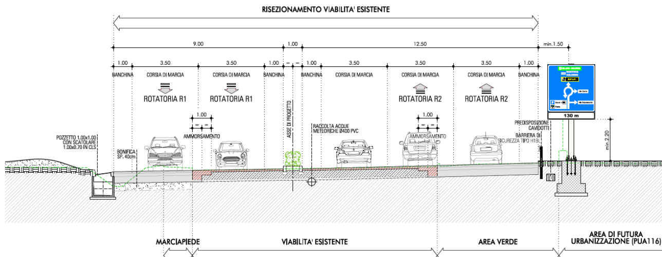
FIGURA 2-2 SEZIONE TIPO TRATTO DI COLLEGAMENTO DA R1 A R2
