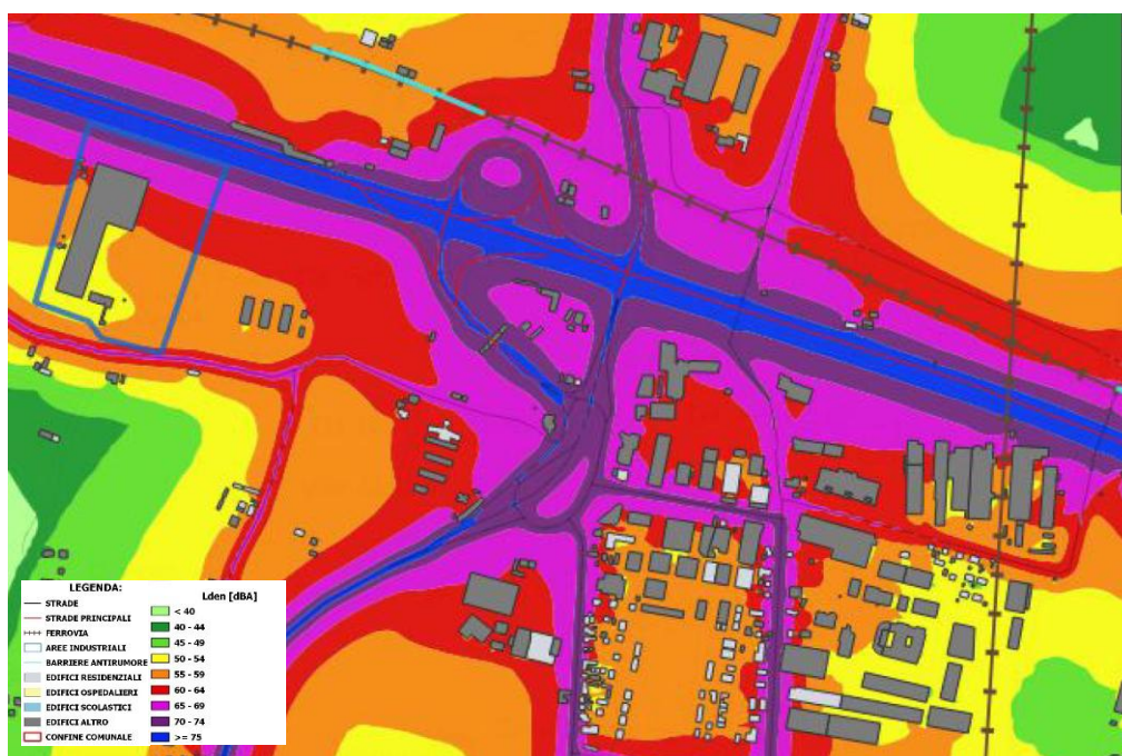
FIGURA 4-13 MAPPATURA ACUSTICA STRATEGICA – L NIGHT
