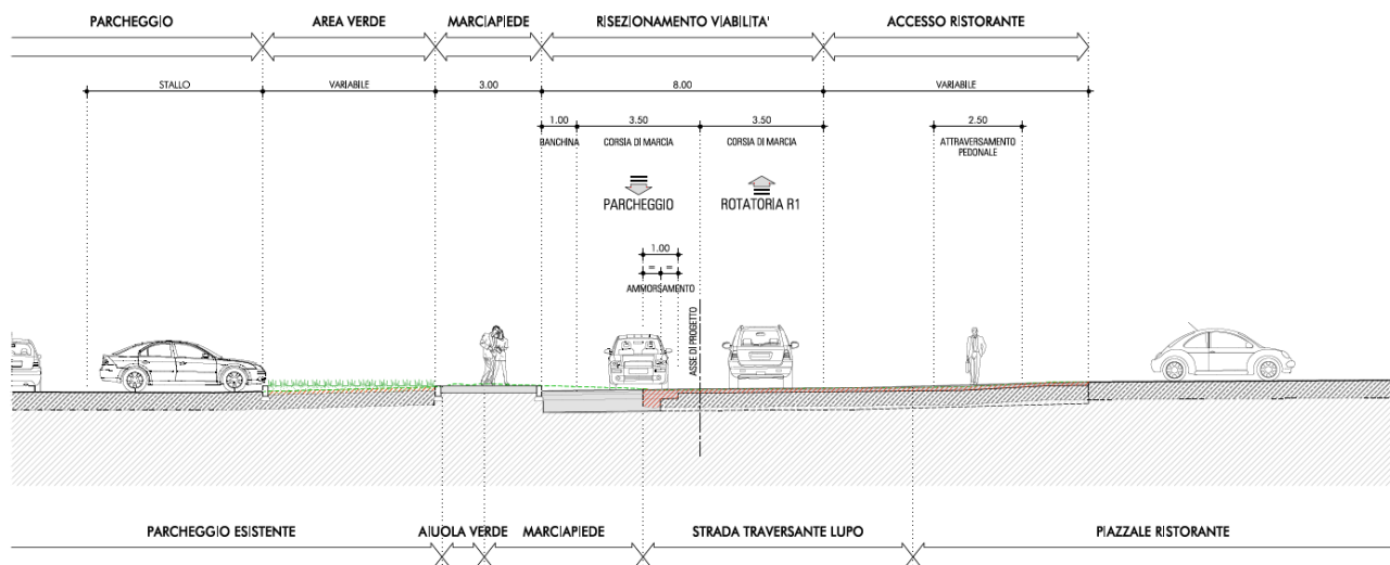
FIGURA 2-6 SEZIONE TIPO RAMO DI COLLEGAMENTO R1 – R3
