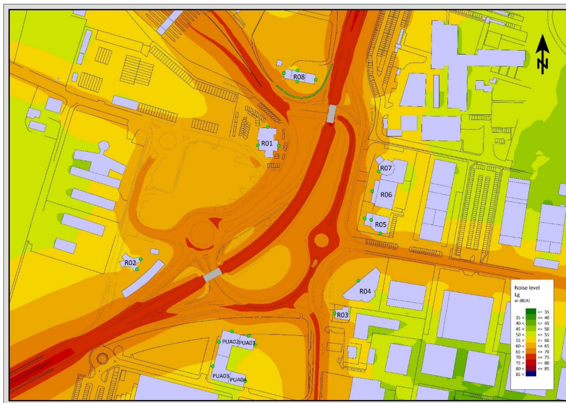
FIGURA 5-5 MAPPATURA ACUSTICA A 4M – POST OPERAM – PERIODO DIURNO
