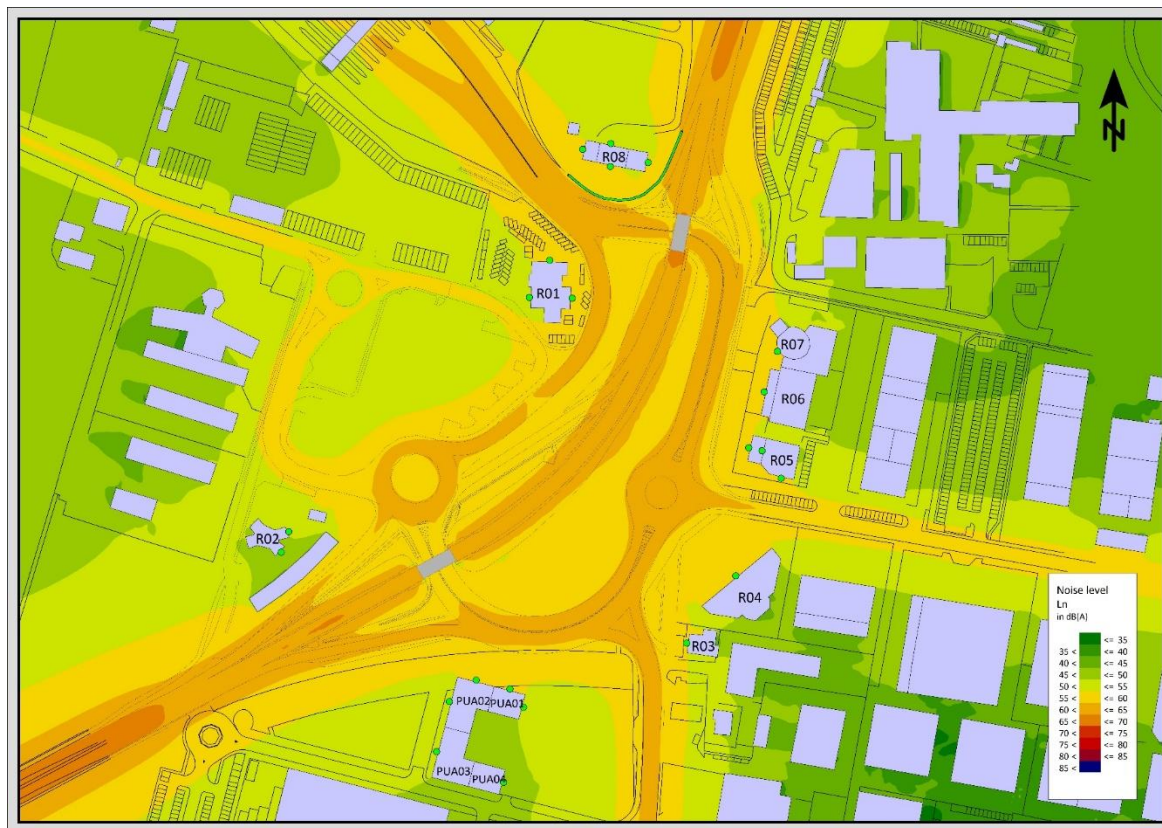
FIGURA 5-6 MAPPATURA ACUSTICA A 4M – POST OPERAM – PERIODO NOTTURNO
