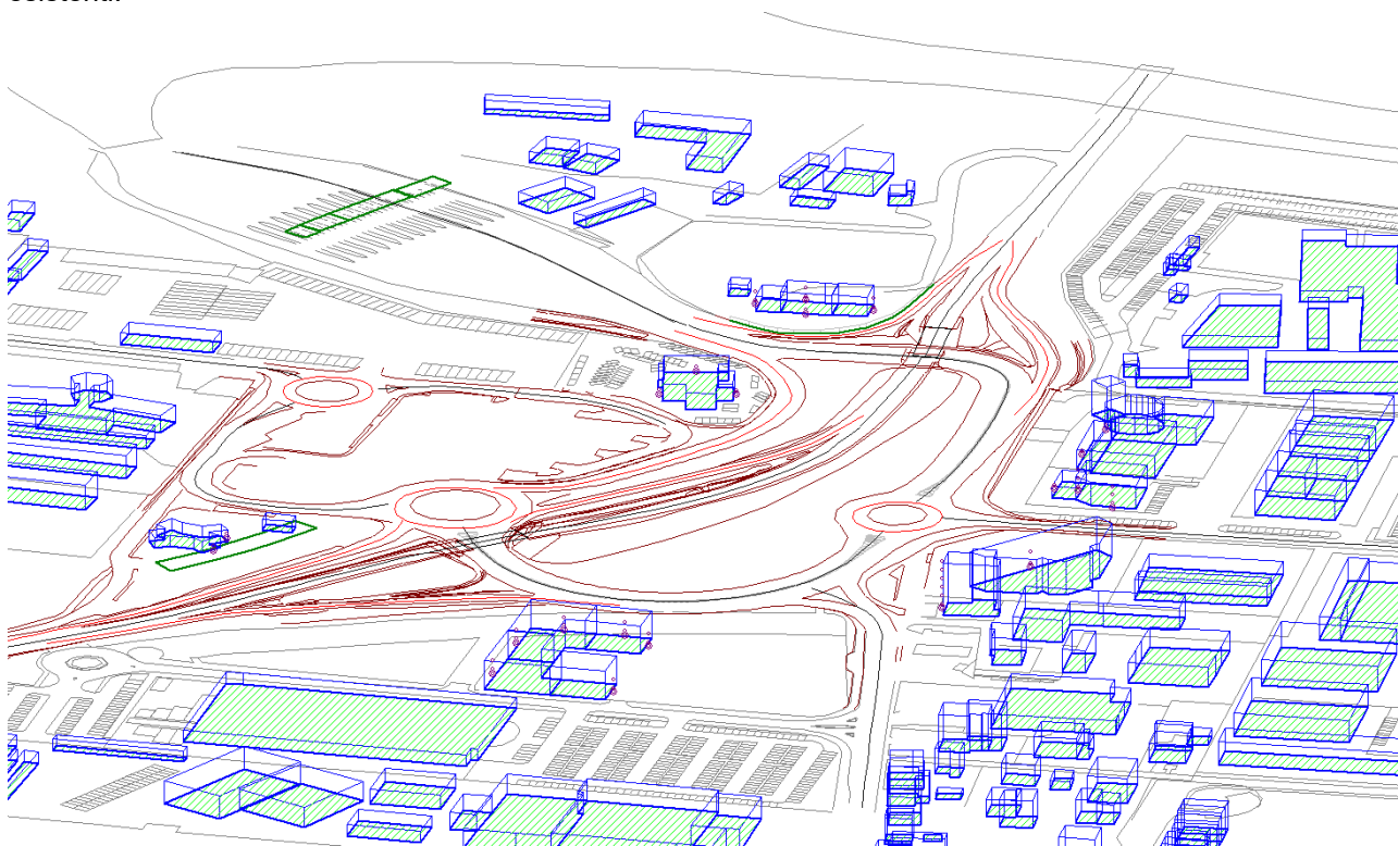
FIGURA 5-4 – STRALCIO 3D DEL MODELLO ACUSTICO
