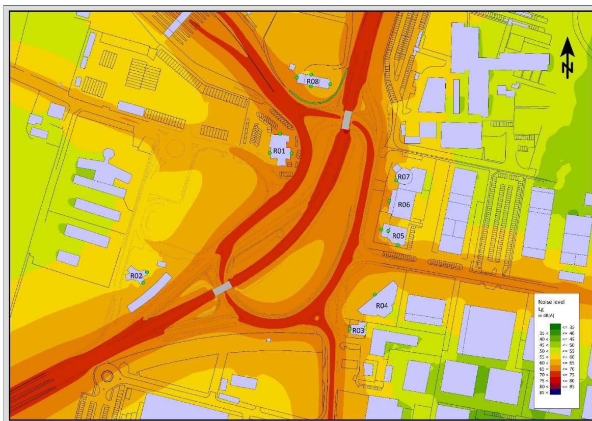
FIGURA 4-15 MAPPATURA ACUSTICA A 4M – ANTE OPERAM – PERIODO DIURNO
