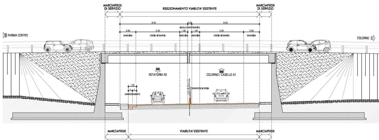
FIGURA 2-3 SEZIONE TIPO IN CORRISPONDENZA DEL CAVALCAVIA SS343 ESISTENTE
