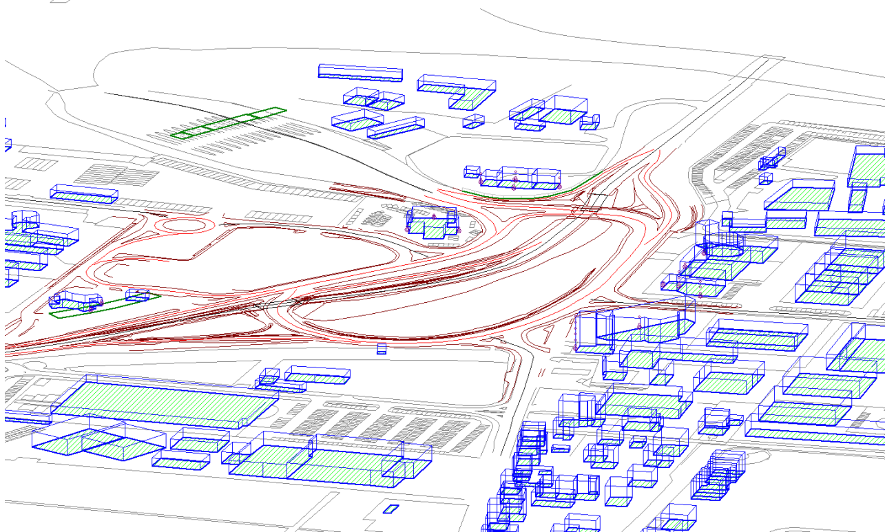
FIGURA 4-14 – STRALCIO 3D DEL MODELLO ACUSTICO
