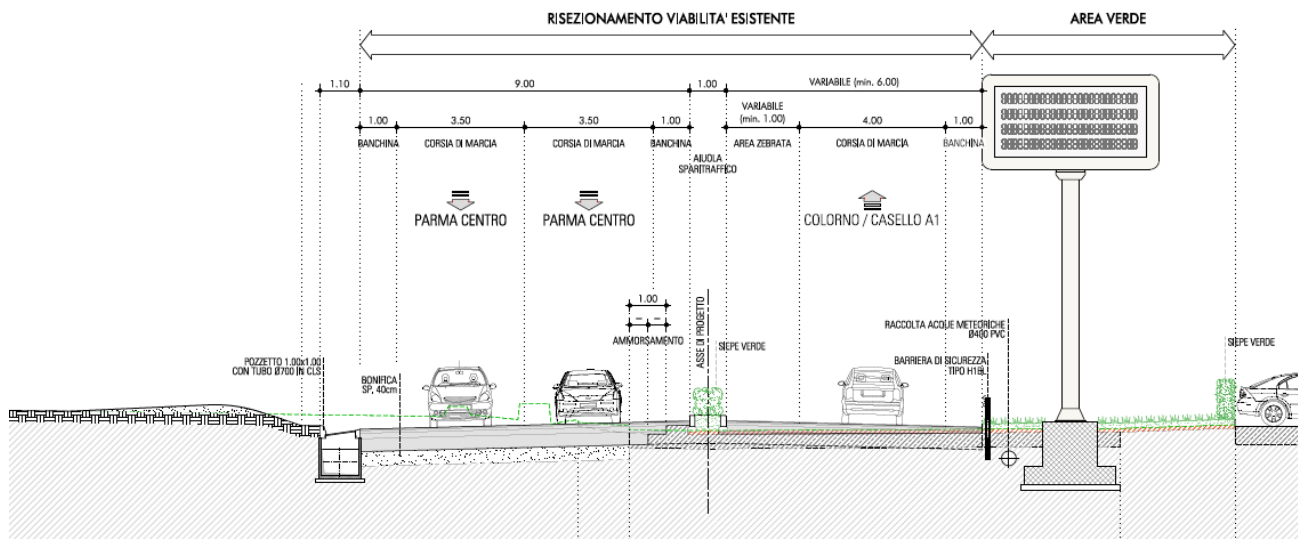
FIGURA 2-4 SEZIONE TIPO TRATTO DI COLLEGAMENTO DA R2 A CASELLO A1
