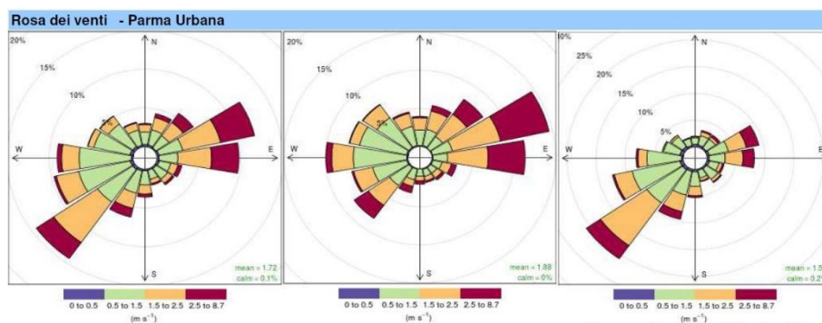
FIGURA 4-4 ROSA DEI VENTI GIORNALIERA, DIURNA E NOTTURNA – PARMA URBANA
