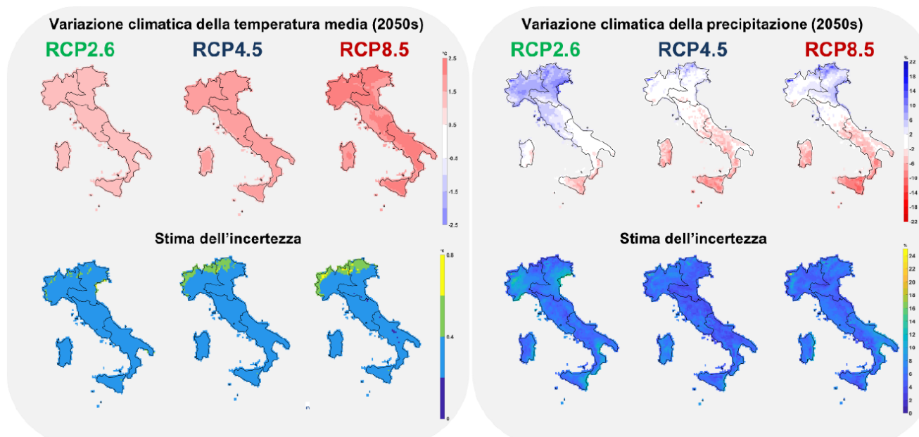
FIGURA 4-6 VARIAZIONI CLIMATICHE ANNUALI DELLE TEMPERATURE MEDIE E DELLE PRECIPITAZIONI CUMULATE MEDIE PER IL PERIODO 2036-2065 (2050s), RISPETTO AL PERIODO DI RIFERIMENTO 1981-2010, PER GLI SCENARI RCP 2.6, RCP 4.5 E RCP8.5
