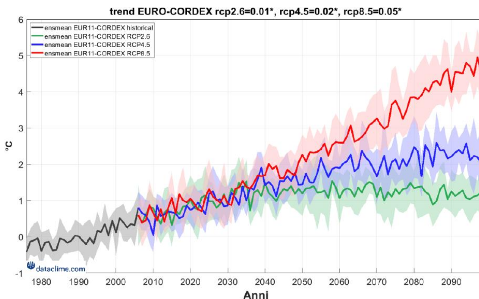
FIGURA 4-5 ANOMALIE ANNUALI DI TEMPERATURA MEDIA (°C) SU SCALA NAZIONALE OTTENUTE A PARTIRE DAI MODELLI EURO-CORDEX
