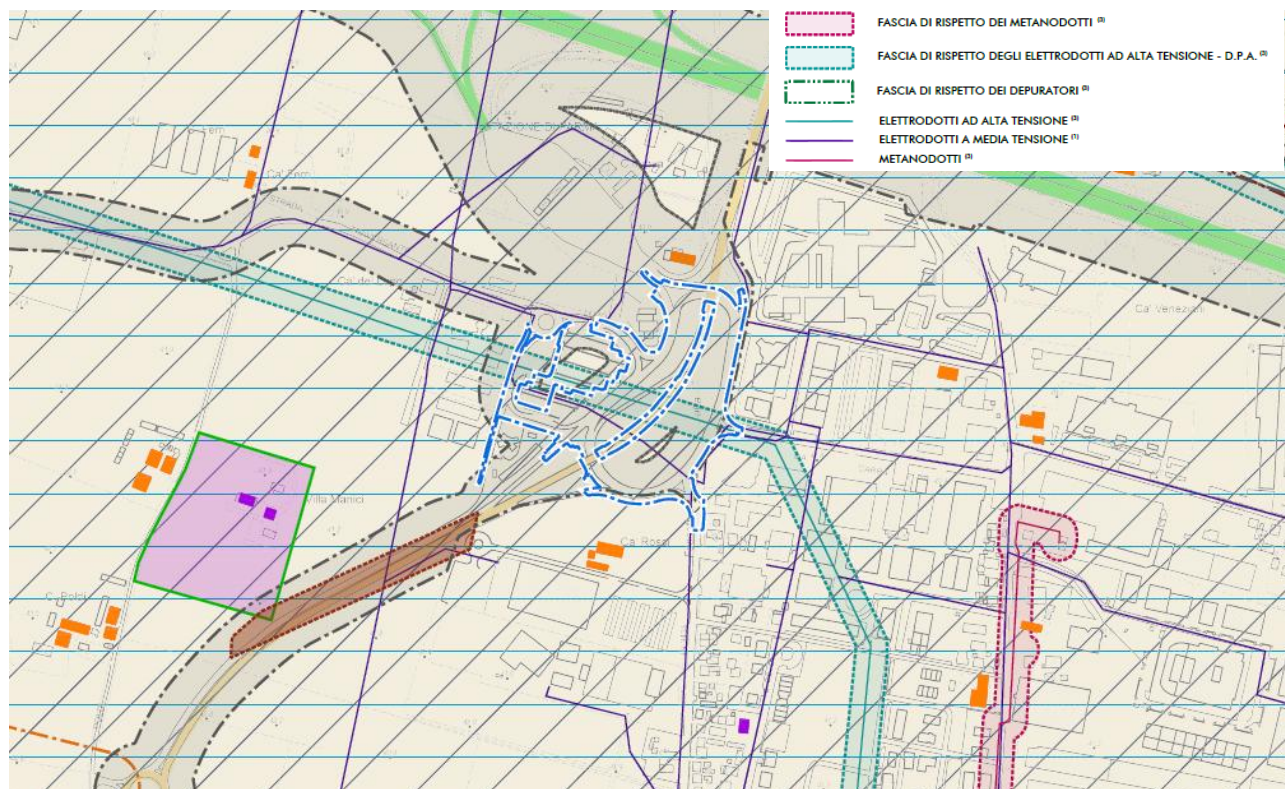
FIGURA 4-17 RETE DI DISTRIBUZIONE E SOTTOSTAZIONI NELL'AREA DI STUDIO (FONTE PIANIFICAZIONE)
