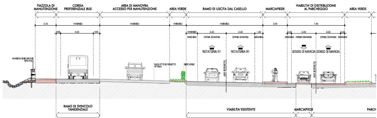
FIGURA 2-5 SEZIONE TIPO RAMO DI USCITA DAL CASELLO A1 E DALLA SS 343
