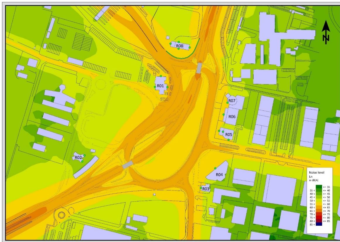
FIGURA 4-16 MAPPATURA ACUSTICA A 4M – ANTE OPERAM – PERIODO NOTTURNO
